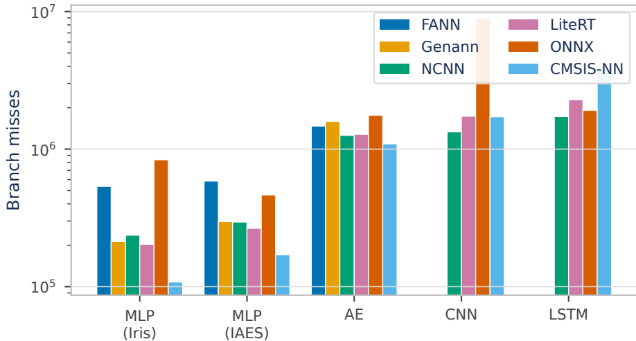
Branch Misses (total por 1000 inferências)
