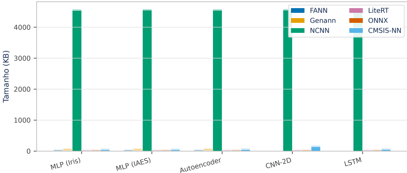
Footprint de memória estática dos executáveis (sólido = .text, transparente = .bss)
