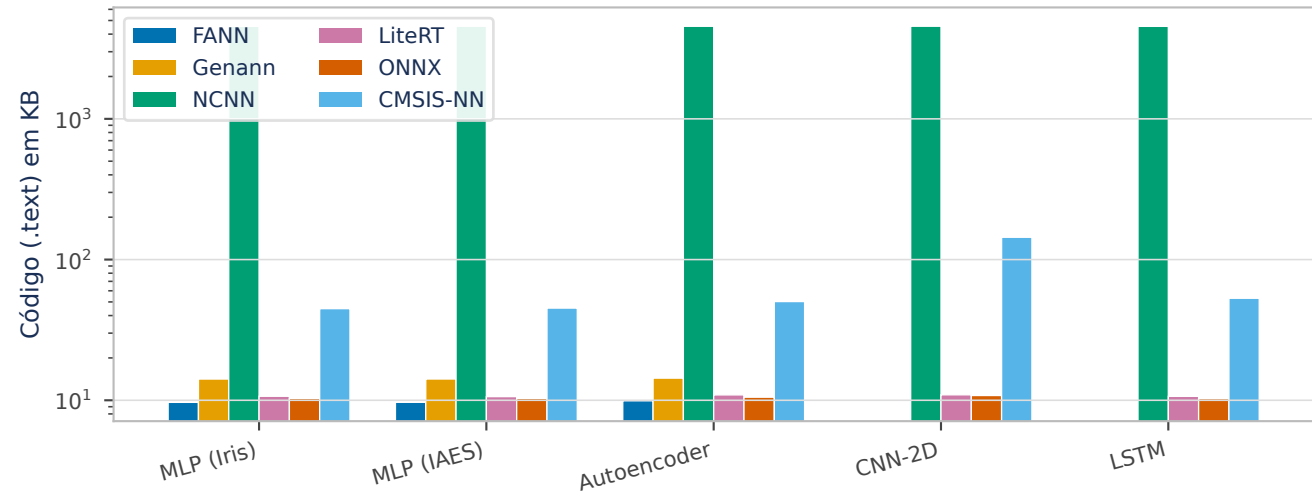
Tamanho do código compilado por framework e algoritmo
