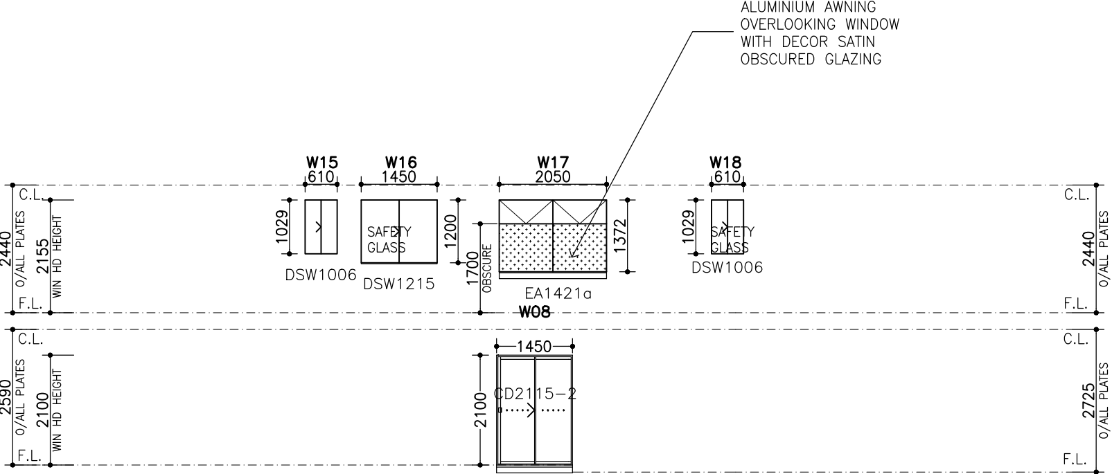
ELEVATION A
