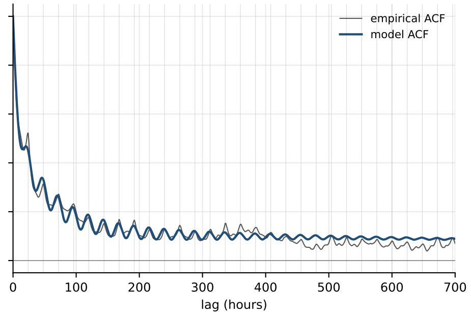
Final CARMA(5,4) QMLE ACF
