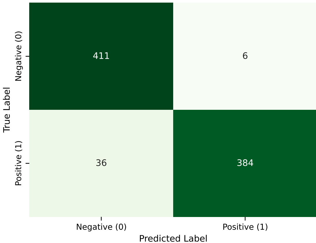
Confusion Matrix - Llama 3.1 CoT-2
