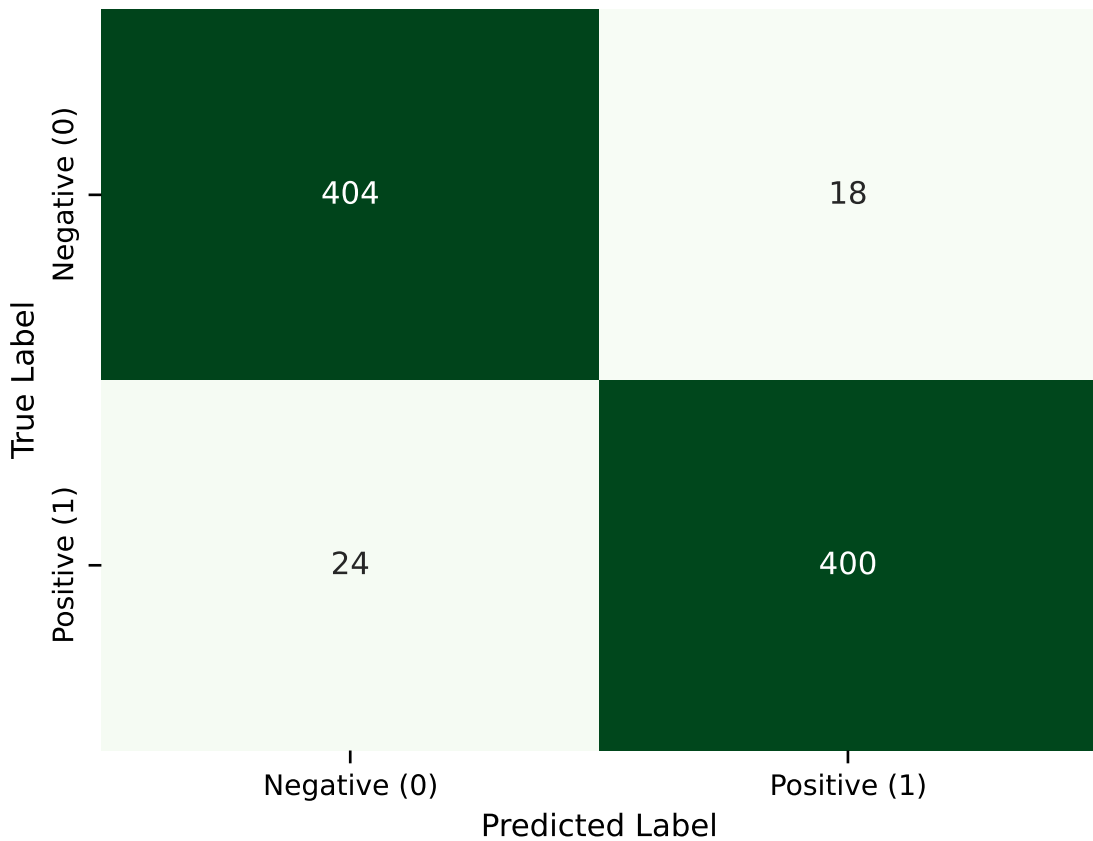
Confusion Matrix - Llama 3.1 CoT-3
