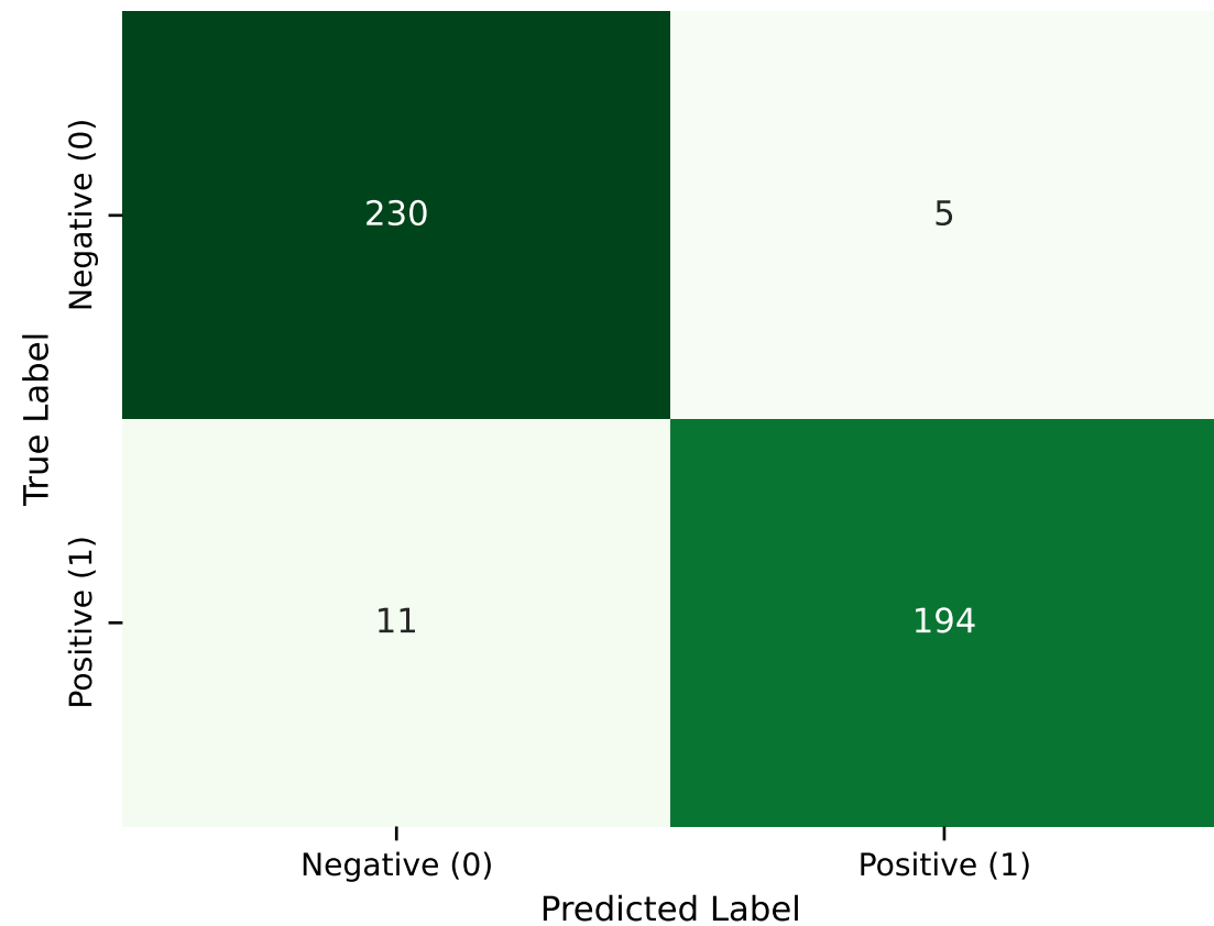
Confusion Matrix - Llama 3.1 FS-2
