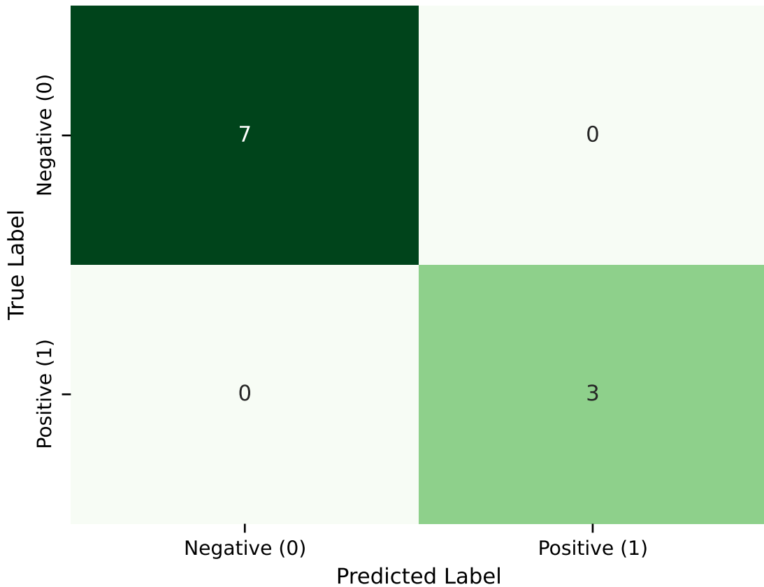
Confusion Matrix - Llama 3.1 ZS-2
