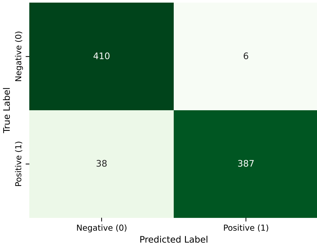
Confusion Matrix - Llama 3.1 ZS-3
