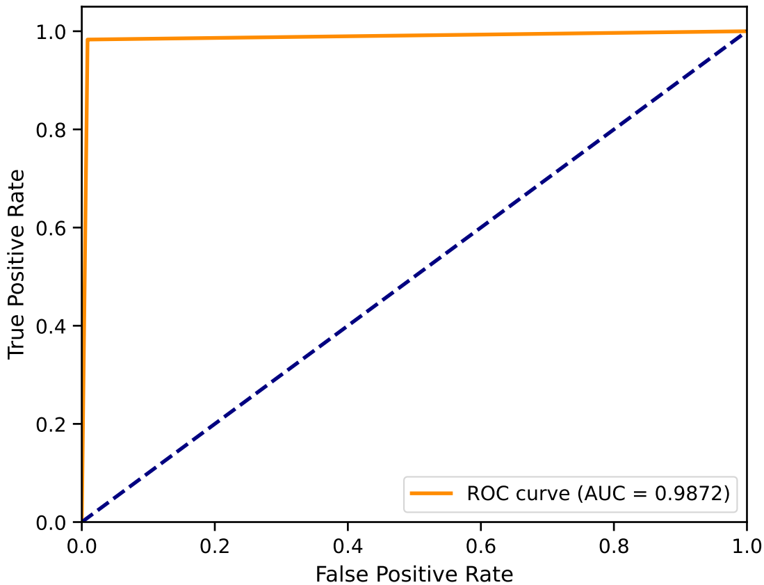
ROC - Llama 3.1 CoT-1
