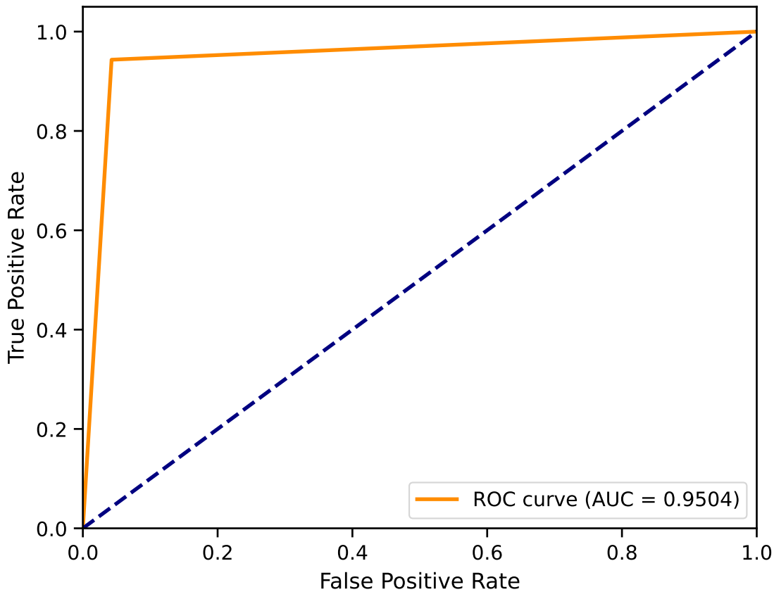
ROC - Llama 3.1 CoT-3
