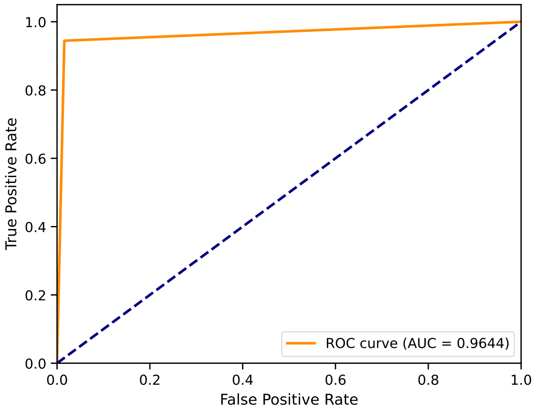
ROC - Llama 3.1 FS-1
