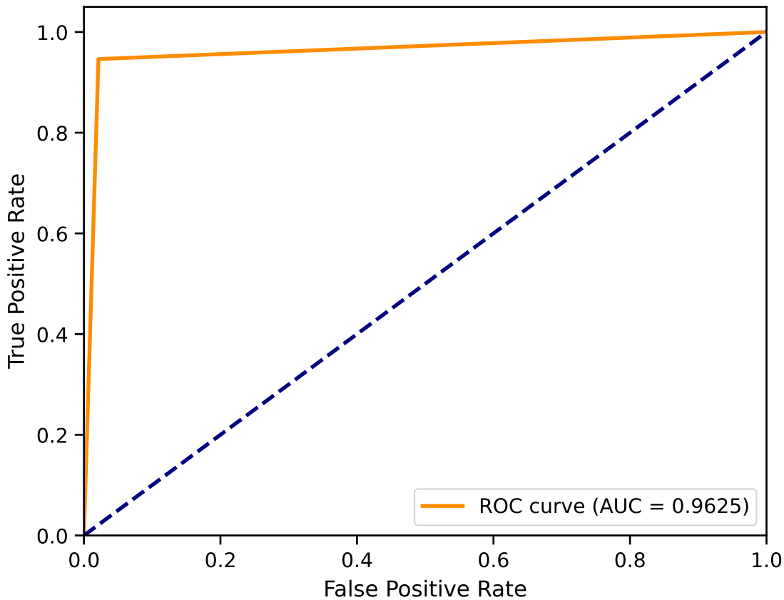
ROC - Llama 3.1 FS-2
