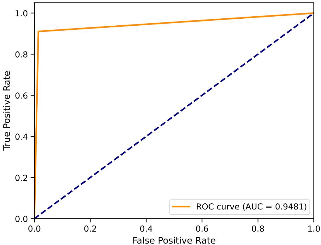
ROC - Llama 3.1 ZS-3
