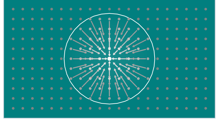
Fig. 3. Representação da estimativa de densidade local a partir das contribuições ponderadas das partículas vizinhas contidas no raio de suporte h .
