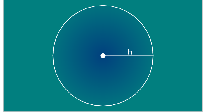
Fig. 2. Representação visual da área de influência (smoothing radius) de uma única partícula central, indicando o decaimento radial da influência do kernel até o raio de suporte h .
