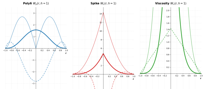
Fig. 3. Os kernels W_\rho , W_s e W_\nu , com h = 1 . As linhas espessas representam os kernels, as finas seus gradientes e as tracejadas o Laplaciano, escalado em 0,1 \times .
