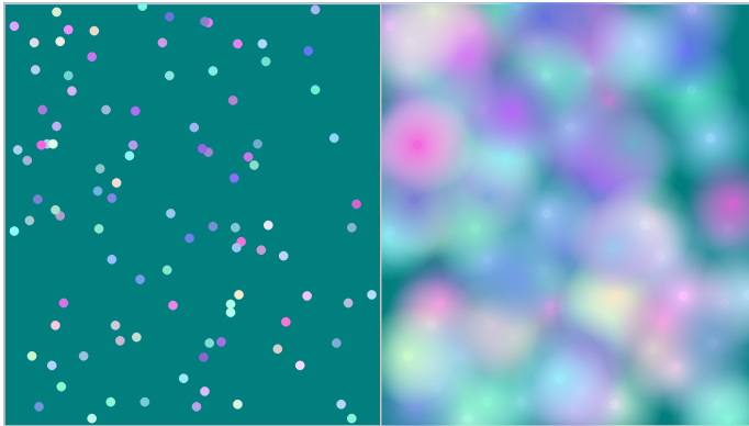
Fig. 1. Mesma distribuição de partículas discretas antes e após a aplicação do kernel de suavização no método SPH.
