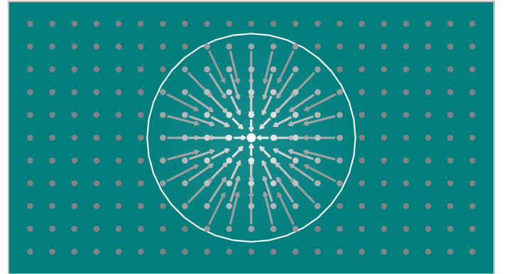
Fig. 4. Representação da visual de densidade local a partir das contribuições ponderadas das partículas vizinhas contidas no raio de suporte h .
