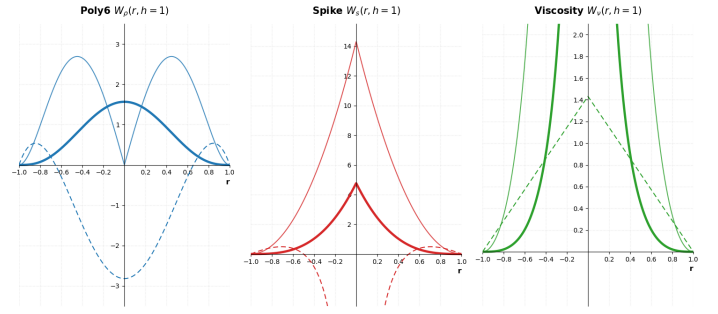
Fig. 3. Os kernels W_\rho , W_s e W_\nu (da esquerda para a direita), com h = 1 em todos os gráficos. As linhas espessas representam os kernels, as finas seus gradientes e as tracejadas o Laplaciano, escalado em 0,1\times .
