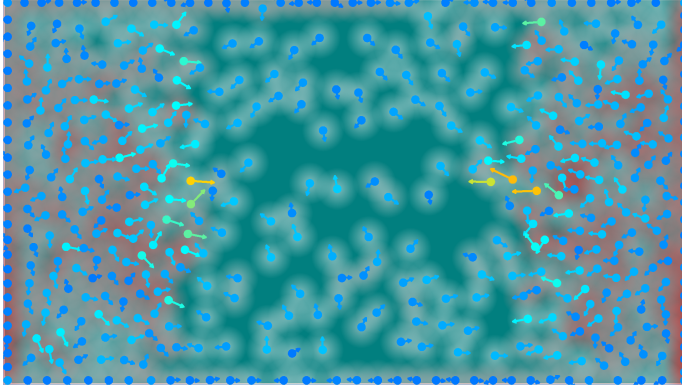
Fig. 6. Representação das forças de pressão entre partículas vizinhas, produzindo aceleração em direção às regiões de menor pressão. Na simulação, as áreas brancas representam a pressão alvo do fluido, enquanto regiões em vermelho indicam alta pressão e em azul representam baixa pressão.
