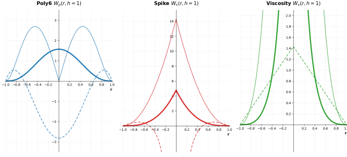
Fig. 4. Os kernels W_\rho , W_s e W_v , com h = 1 . As linhas espessas representam os kernels, as finas seus gradientes e as tracejadas o Laplaciano, escalado em 0,1 \times .
