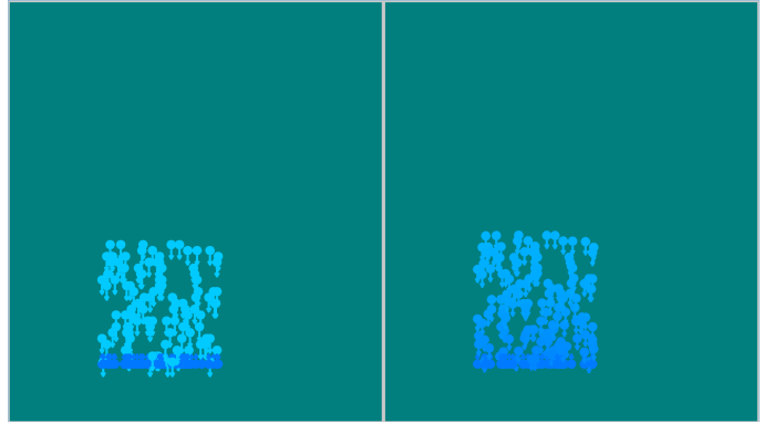
Fig. 7. Representação do efeito viscoso no método SPH. A viscosidade suaviza diferenças locais de velocidade entre partículas vizinhas, produzindo um escoamento mais contínuo e estável.
