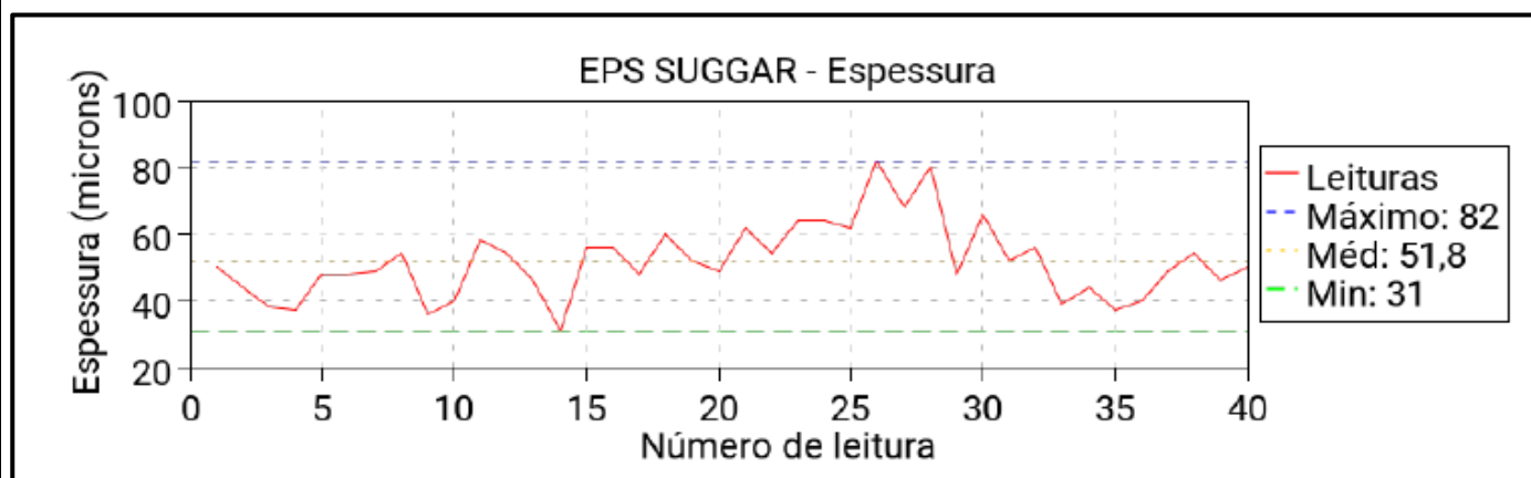
Imagens 16, 17, 18, 19, 20, 21, e 22: Registro fotográfico inspeção da espessura da película seca (média 51µm).
