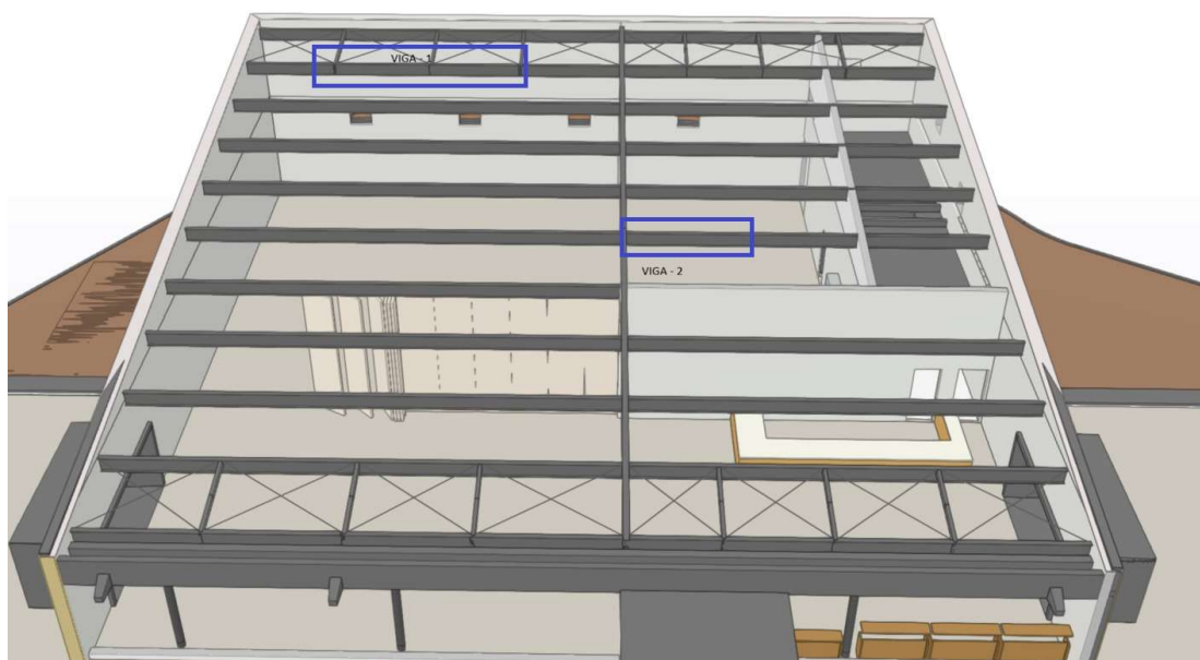
Identificação das vigas 1 e 2 e faces que foram realizadas as medições.
