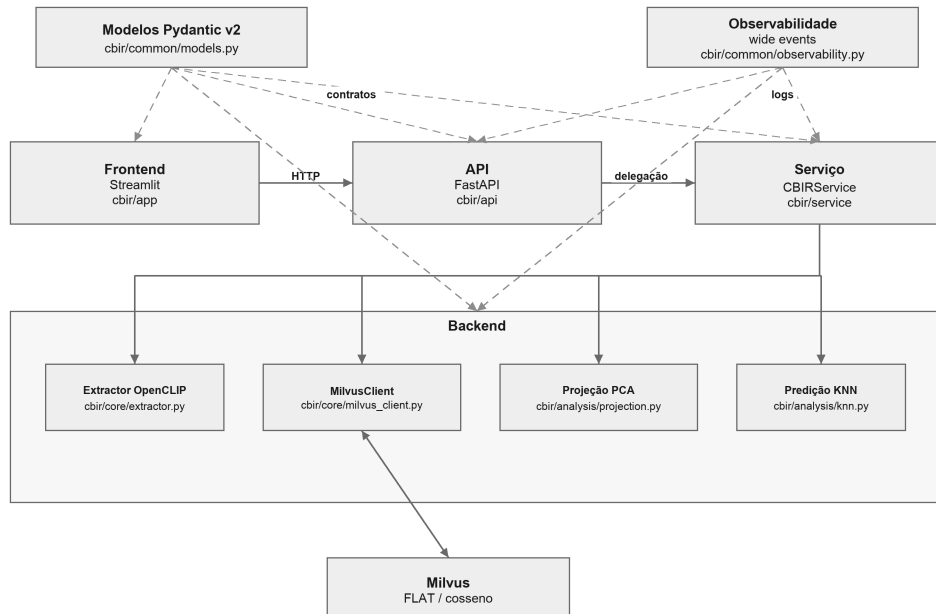
Figura 1: Arquitetura em três camadas. O frontend fala apenas com a API; a API delega ao serviço; o serviço orquestra o backend e o Milvus.
