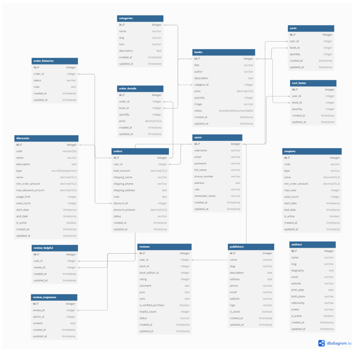
Hình 2.4 : Sơ đồ quan hệ Relationship ERD.
