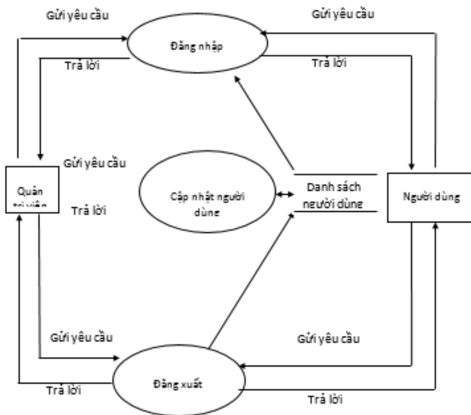
Hình 2.3.3.1: Hình biểu đồ luồng dữ liệu mức đỉnh chức năng quản trị .
