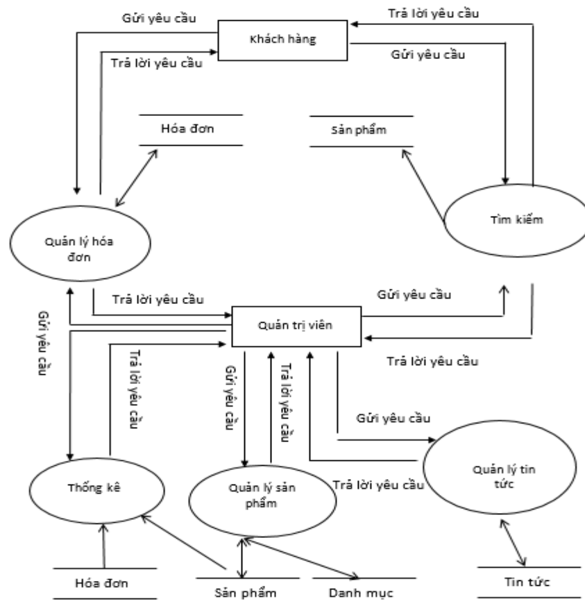
Hình 2. 3.2: Hình biểu đồ luồng dữ liệu mức đỉnh.
