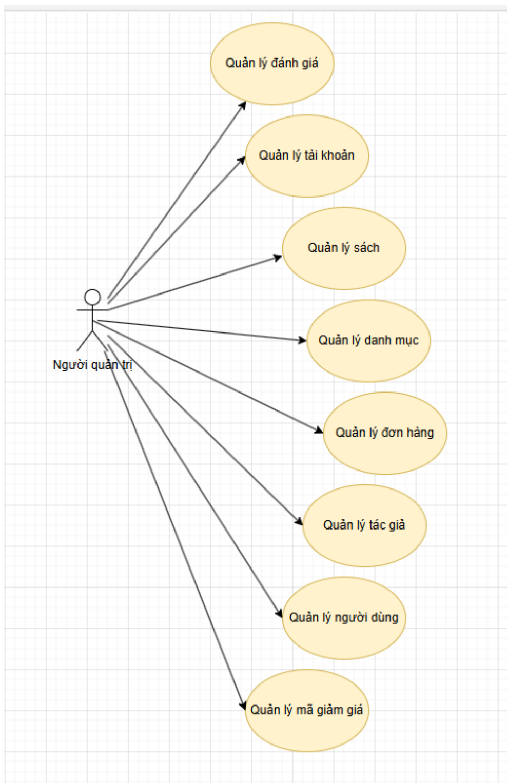
Biểu đồ 2.2.3.1. : biểu đồ tổng quan use case quản trị.
