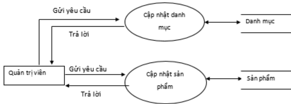
Hình 2.3.4.1 : Hình Biểu đồ luồng dữ liệu mức dưới đỉnh chức năng “Quản lý sản phẩm”.
