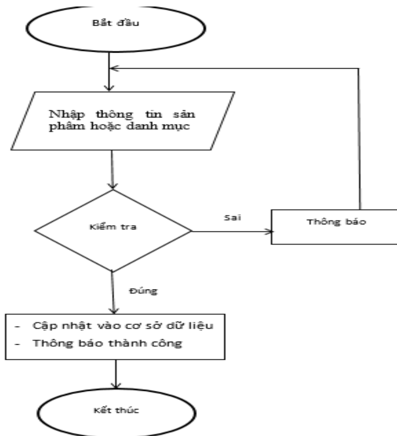
Hình 2.3.4.2 : Hình lưu đồ thuật toán đặc tả chức năng quản lý sản phẩm .
