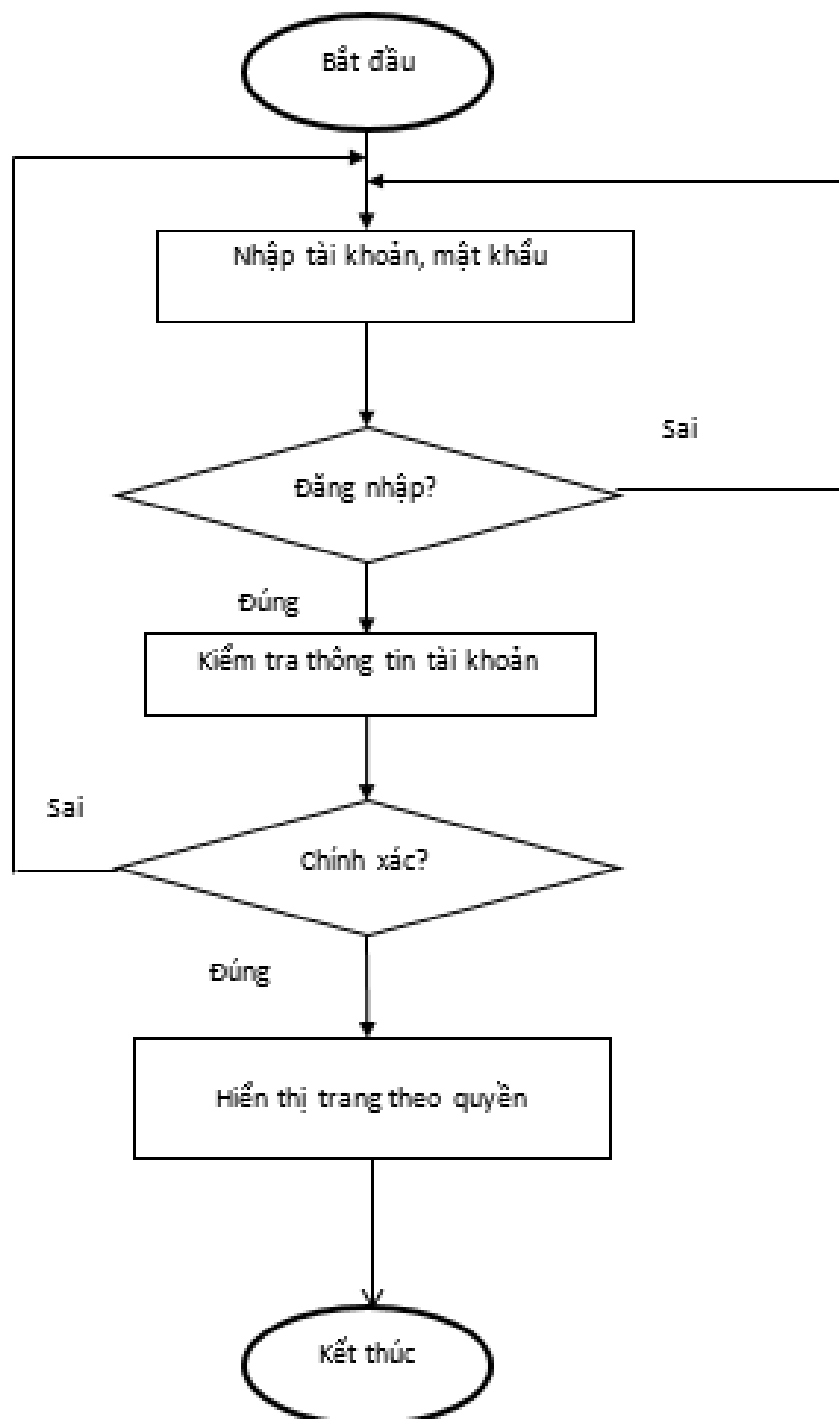
Hình2.3.3.2 : Hình sơ đồ khối đặc tả chức năng đăng nhập .
