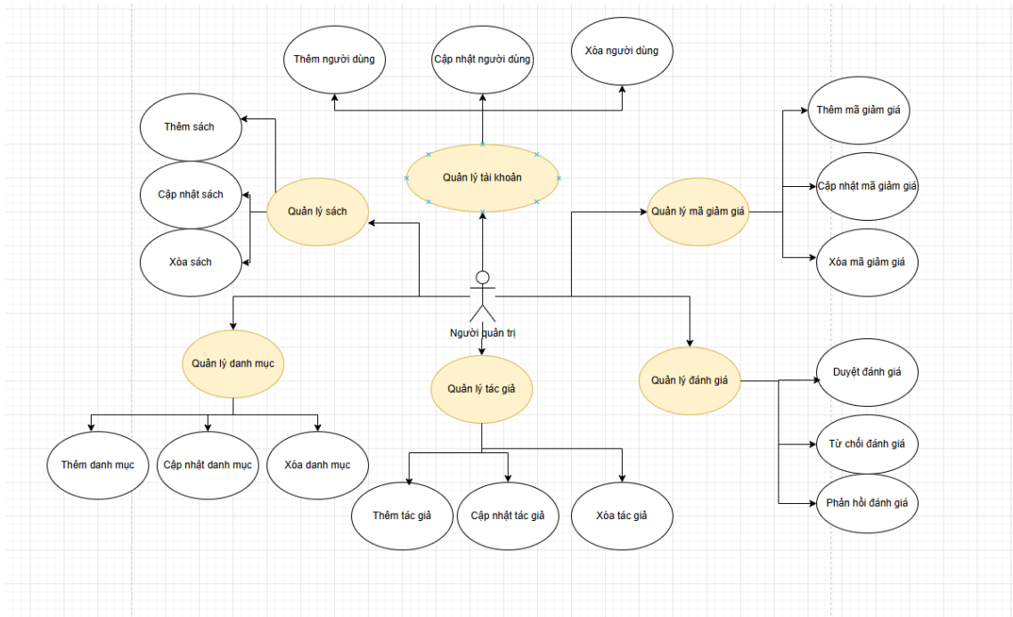
Biểu đồ 2.2.3.2. : Biểu đồ phân tách chức năng.
