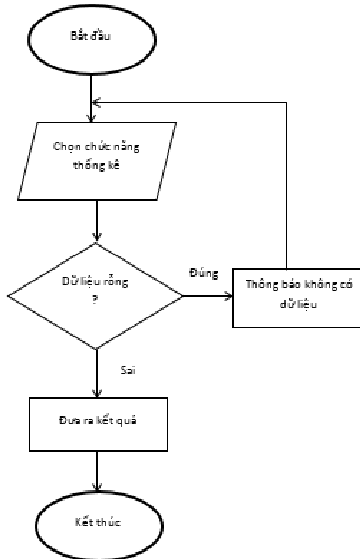
Hình 2.3.9.2 : Lưu đồ thuật toán đặc tả chức năng thống kê .
