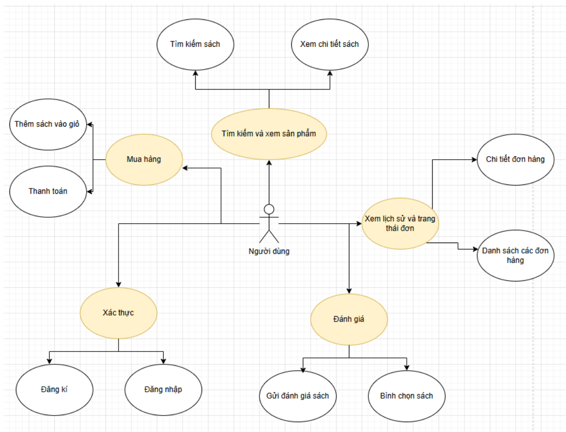
Biểu đồ 2.2.2.2 : Biểu đồ phân tách chức năng.
