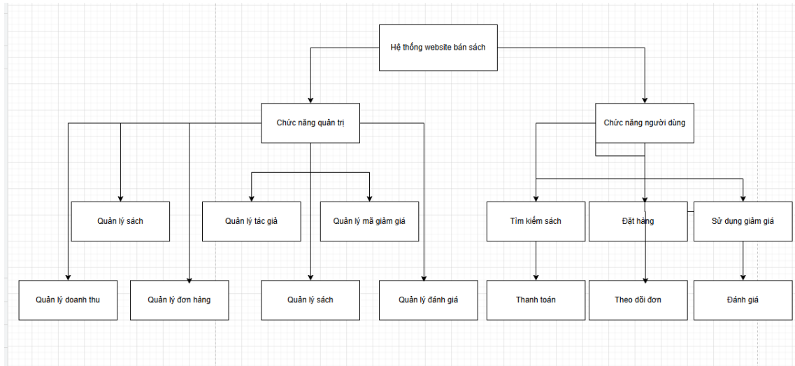
Sơ đồ 2.1: sơ đồ phân rã chức năng .
