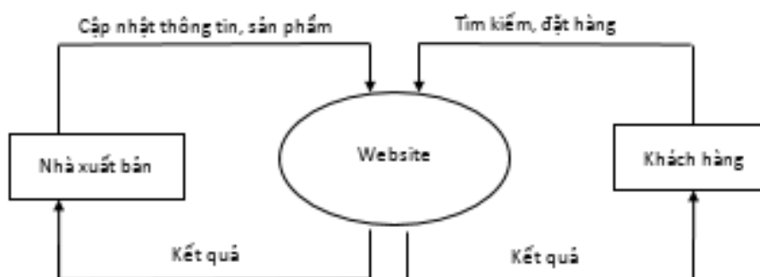
Hình 2.3.1: Hình biểu đồ luồng dữ liệu ngữ cảnh.
