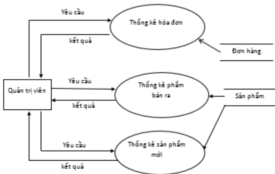
Hình 2.3.8. Biểu đồ luồng dữ liệu mức dưới đỉnh chức năng “Thống kê”.
