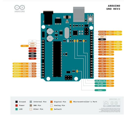
Fig. 4. Arduino Pinout
