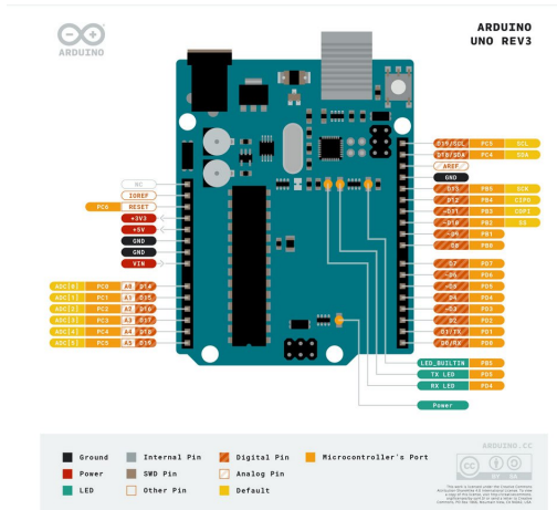
Fig. 4. Arduino Pinout
