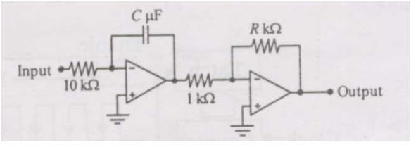
Fig. 1.1.56.1
