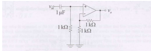
Fig. 1.1.135.1
