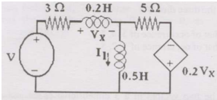
Fig. 1.1.40.1
