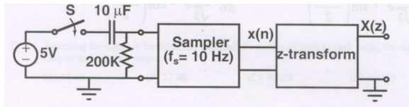
Fig. 1.2.92.1
