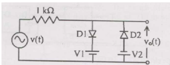
Fig. 1.1.67.1
