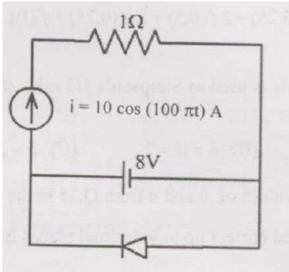
Fig. 1.1.66.1
