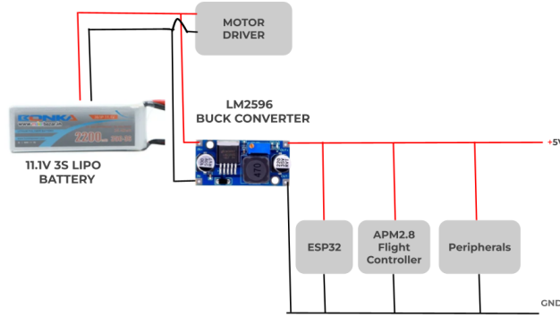
Fig. 3: Power distribution visualisation
