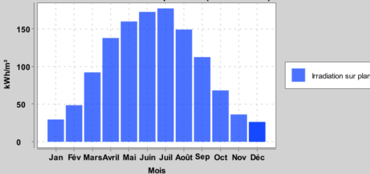
Irradiation mensuelle sur plan fixe (kWh/m 2 /mois)
