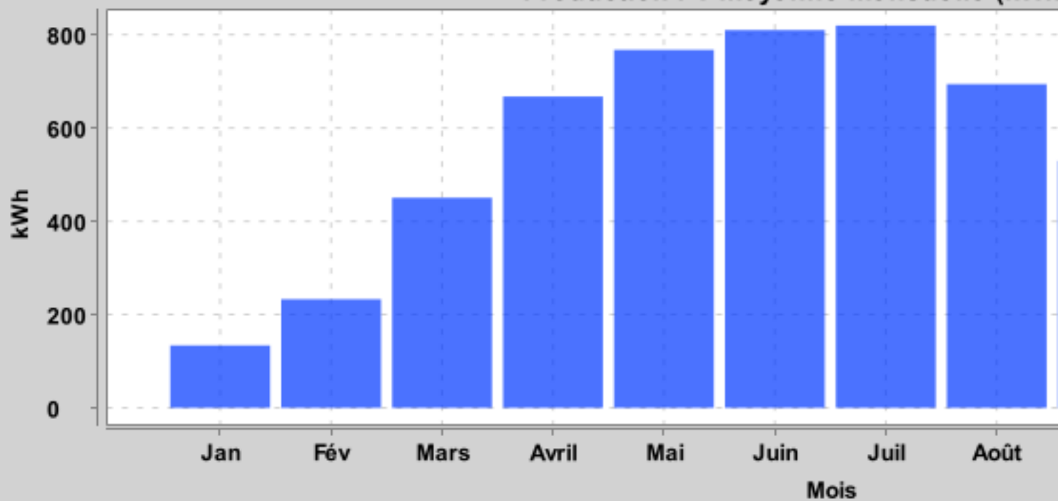
Production PV moyenne mensuelle (kWh)
