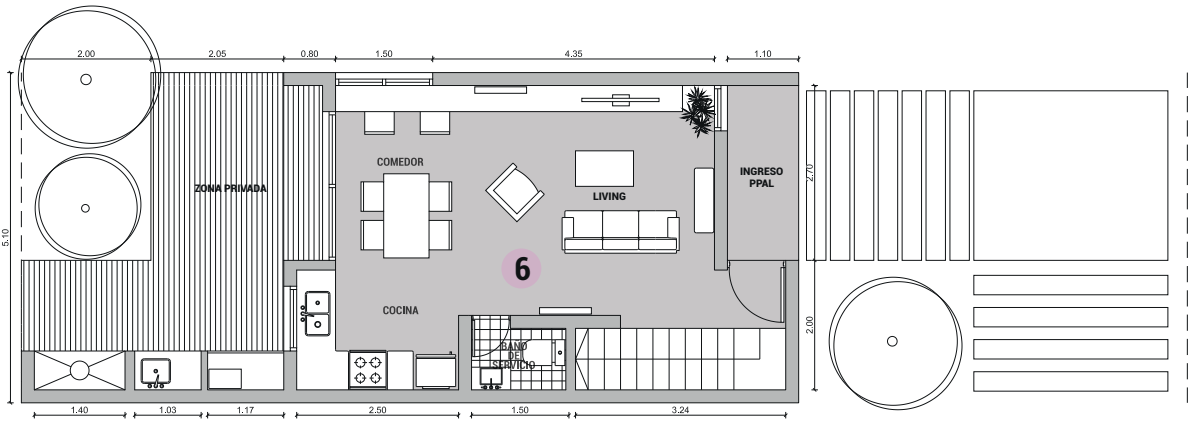
TIPOLOGÍA 3 M2 CUBIERTO Y SEMICUBIERTO
