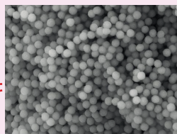
Imagen SEM de PALFIQUE OMNICHROMA con un aumento de 20.000X
