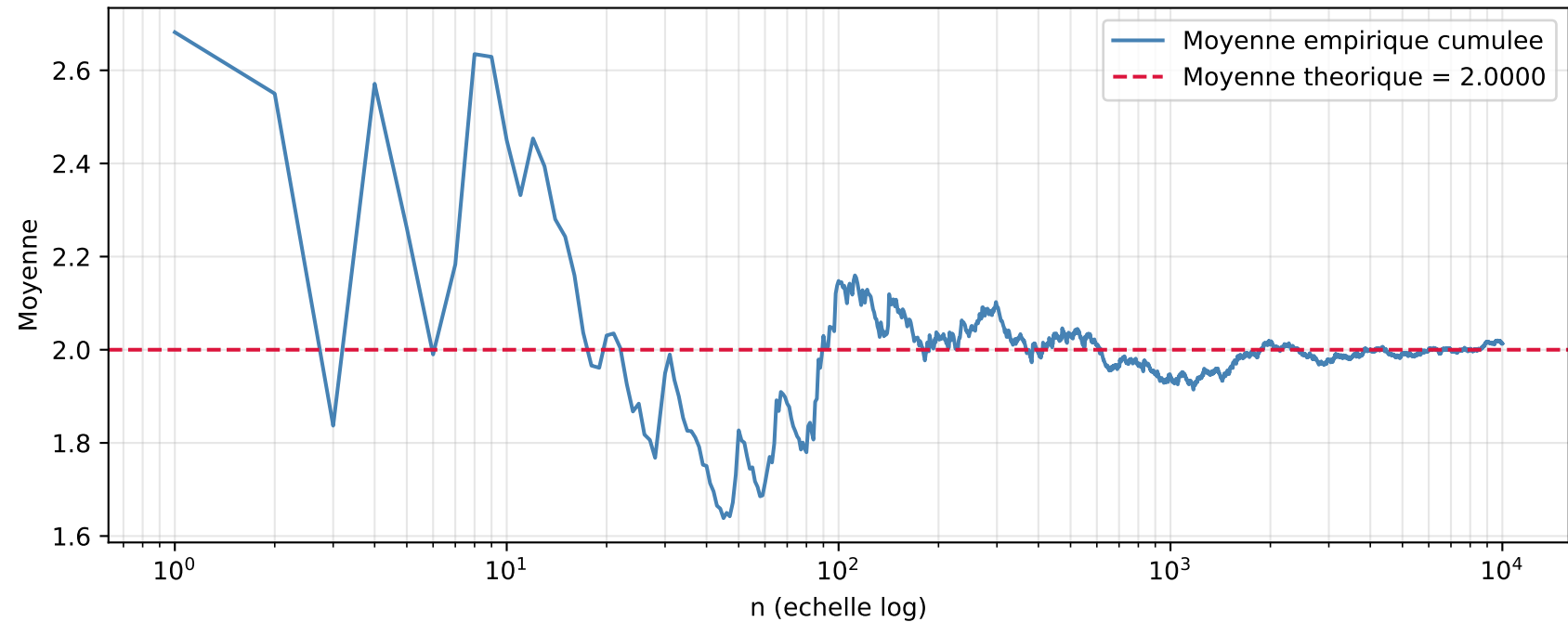
Convergence de la moyenne empirique - exponentielle
