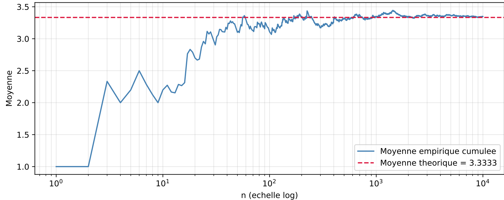
Convergence de la moyenne empirique - geometrique
