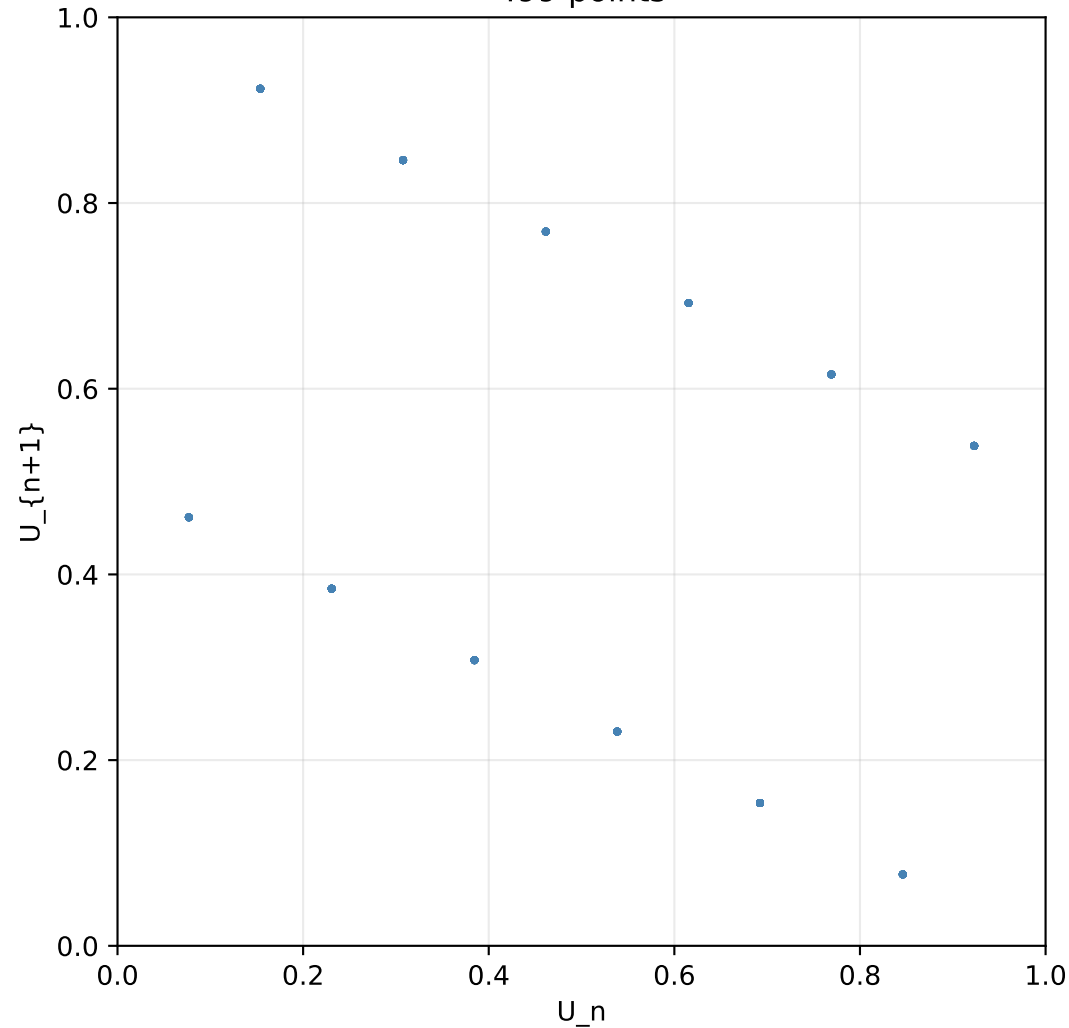
Paires ( U_n , U_{n+1} ) - Multiplicatif court ( a=6 , m=13 ) 499 points
