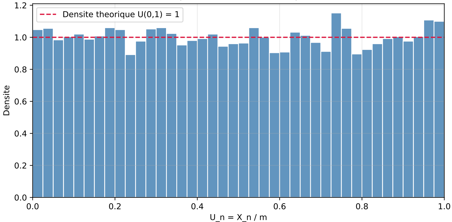
Distribution des U_n produits par : MINSTD (Park-Miller) ( n = 10000 échantillons)
