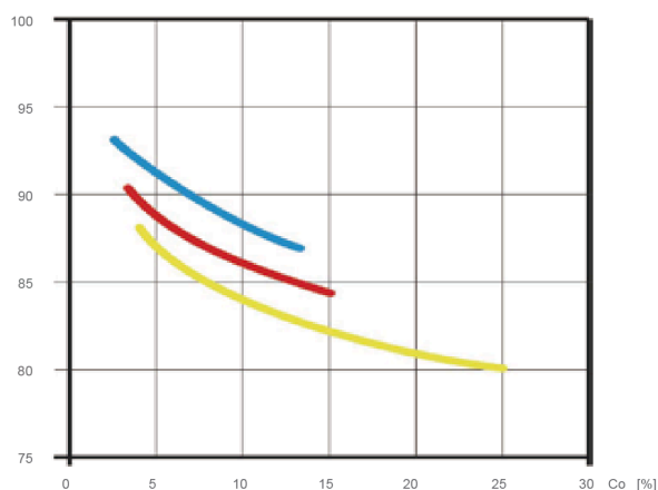
Твёрдость по Роквеллу, HRA
