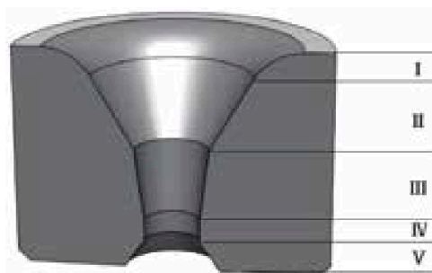
Разрез волокни: пять функциональных зон канала
