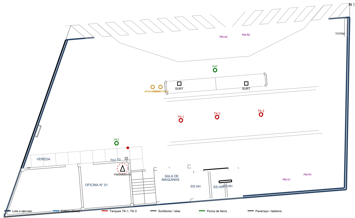
Figura 9.1: Vista esquematica de la geometria base extraida del plano original CAD-002 (reconstruccion academica de layout-grifo.json). Los limites de areas y las cotas deben verificarse en campo.
