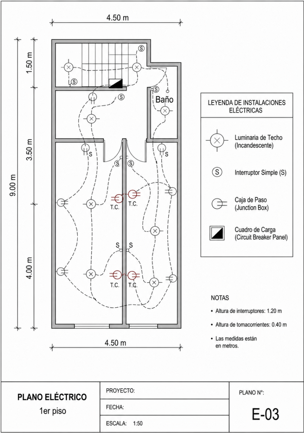
Figura 7.1: Plano de Instalaciones Eléctricas - Primer Piso
