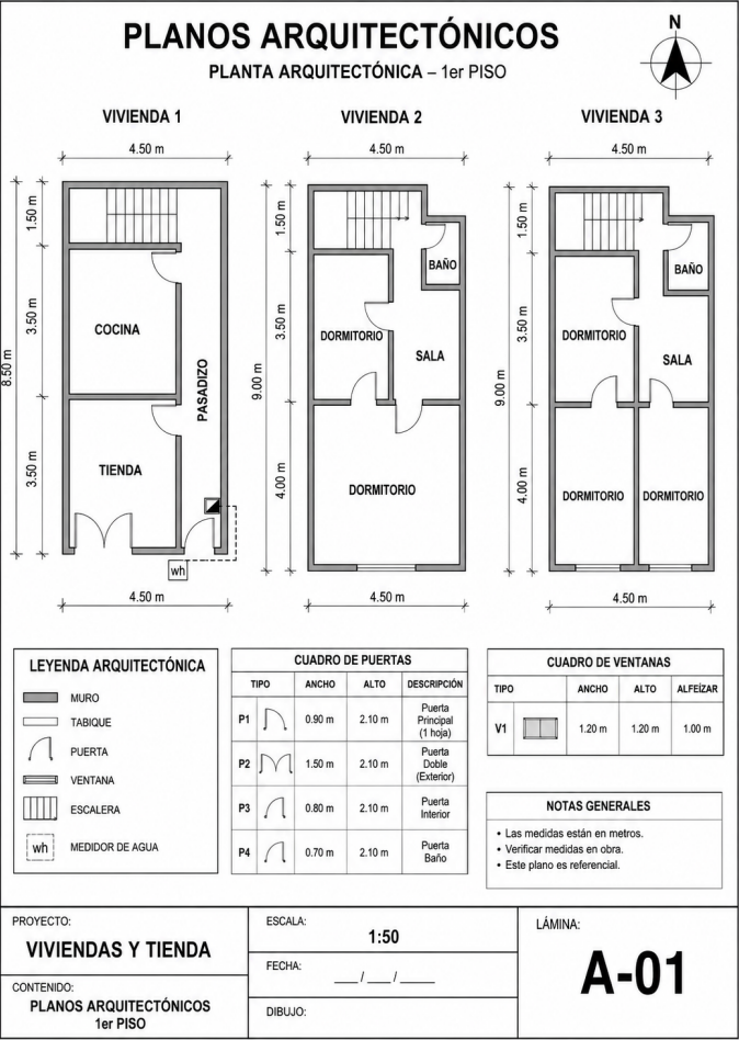
Figura 7.4: Plano Arquitectónico General
