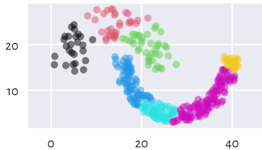
Genie (n_clusters=7)
