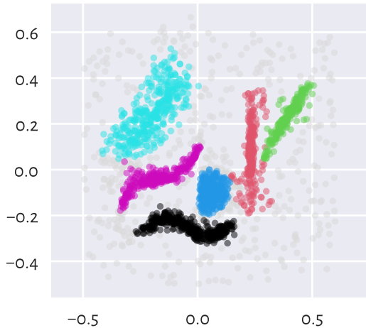
(gini_threshold=0.3, M=25)
