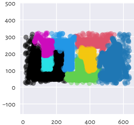
(n_clusters=8)
