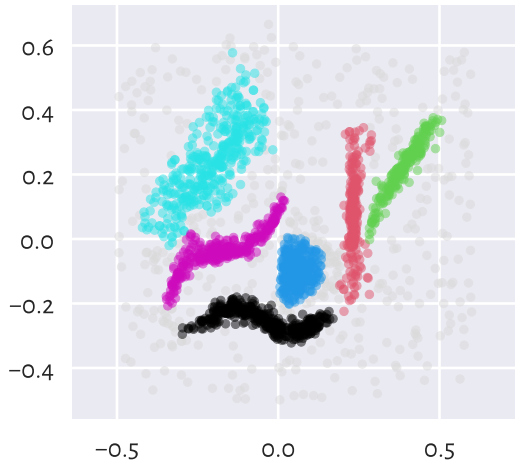
(gini_threshold=0.3, M=10)
