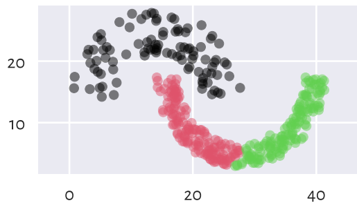
Genie (n_clusters=3)
