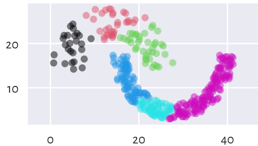
Genie (n_clusters=6)
