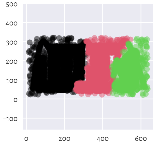
(n_clusters=3)
