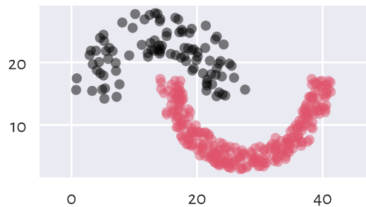
Genie (n_clusters=2)
