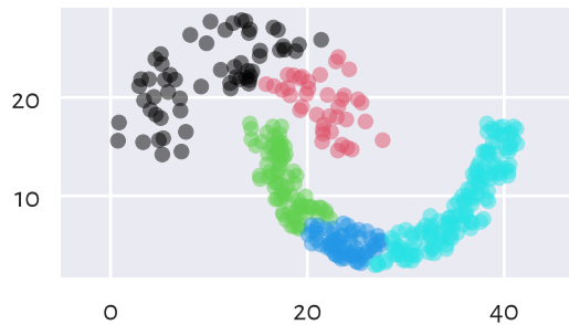
Genie (n_clusters=5)
