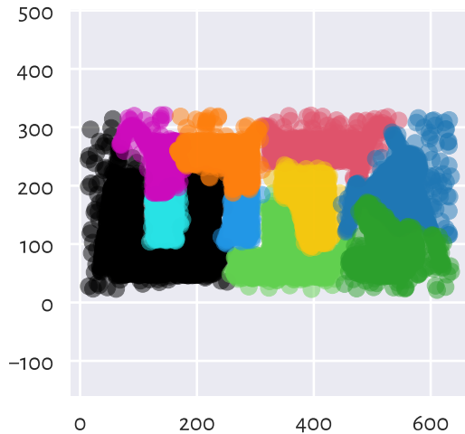
(n_clusters=10)
