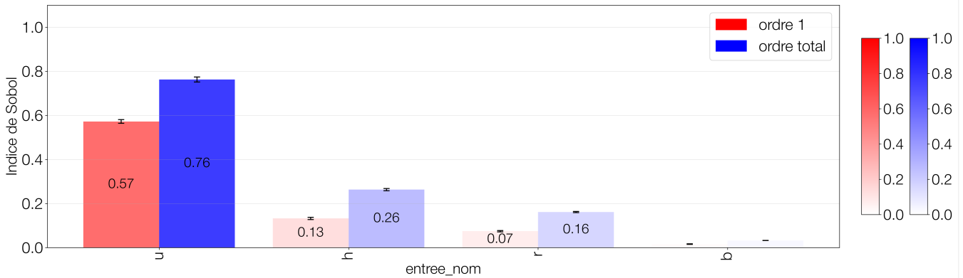
Graphique des barres de Sobol, pour générateur = sobol :
