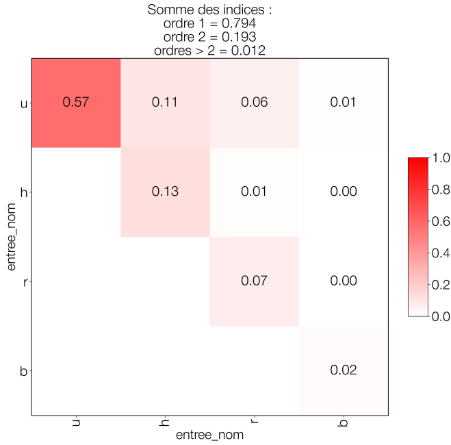
Graphique des matrices de Sobol, pour générateur = sobol :
