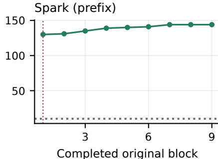
Spark (prefix)
