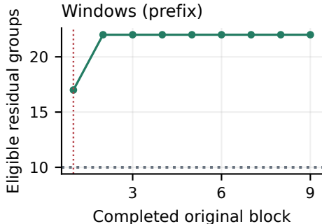
Windows (prefix)
