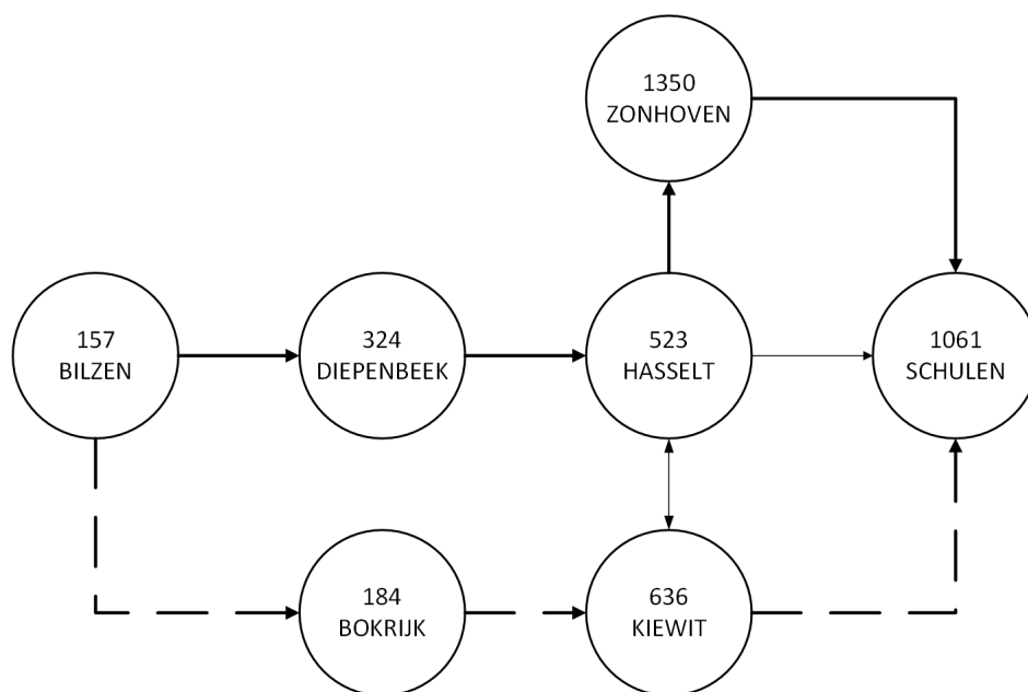
Obrázek 8: Podgraf reprezentující výsledek dotazu 1.
