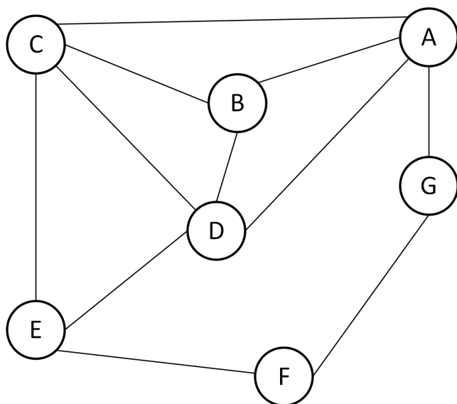
Obrázek 10: Graf pro, který počítáme výskyt trojúhelníků
