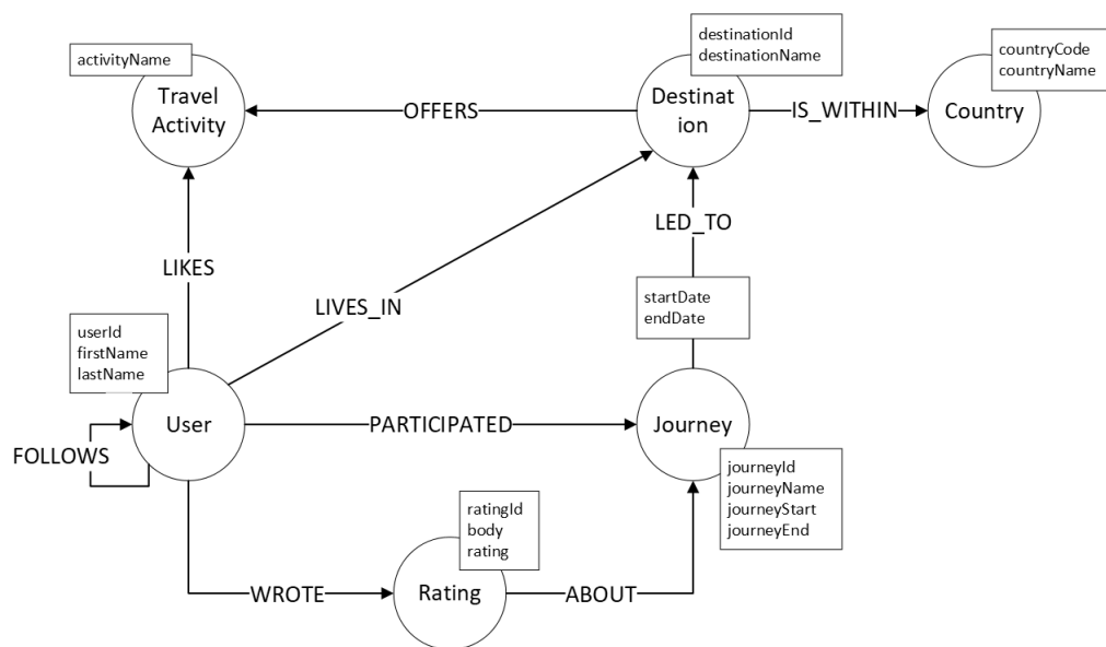
Obrázek 5: Logický datový model pro sociální síť pro cestovní nadšence
