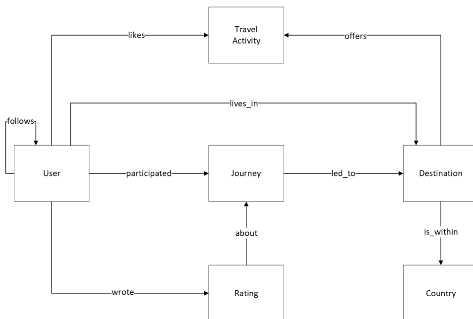
Obrázek 3: Konceptuální datový model pro sociální síť pro cestovní nadšence
