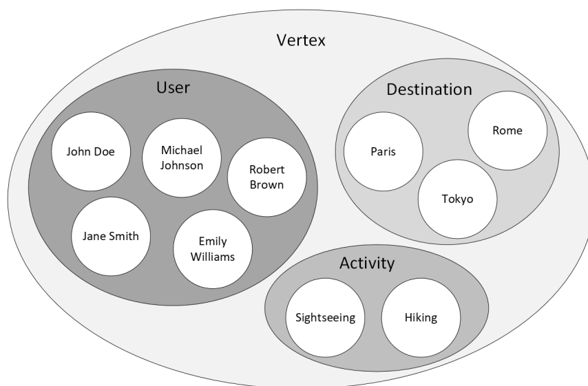
Obrázek 4: Label vrcholu definuje do které kategorie vrchol spadá
