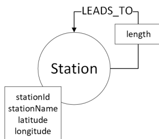
Obrázek 6: Model grafové databáze pro ukázkové příklady v této kapitole
