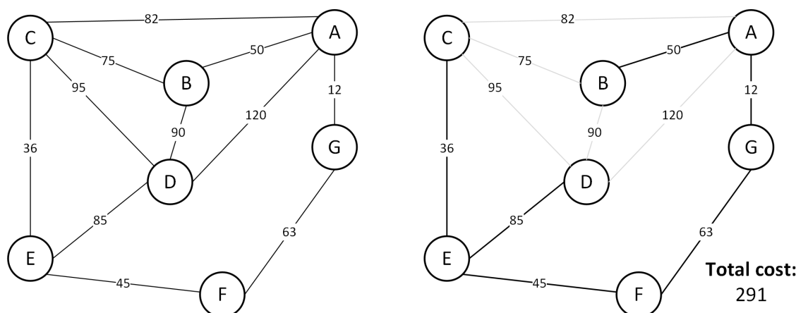
Obrázek 9: Minimální kostra grafu
