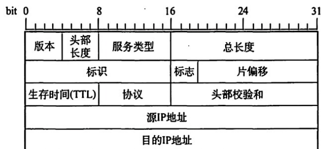
题 47-a 图 IP 分组头结构
