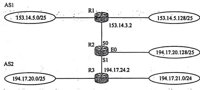
题 47 图 网络拓扑结构
