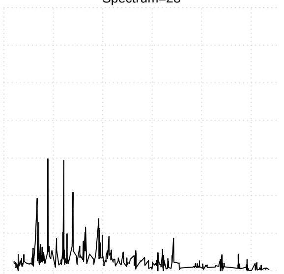
Spectrum=24
