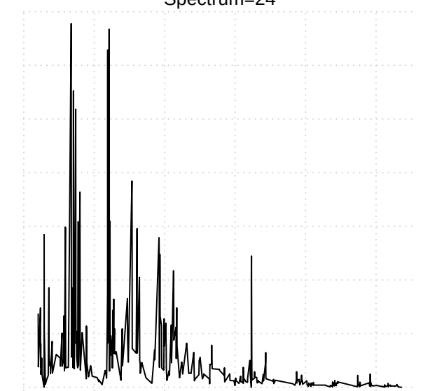
Spectrum=24
