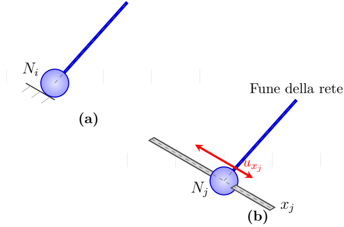
Figura 4.1: Vincoli cinematici: (a) - Cerniera fissa (spostamenti impediti), (b) - Cerniera scorrevole (scorrimento lungo x_j )
