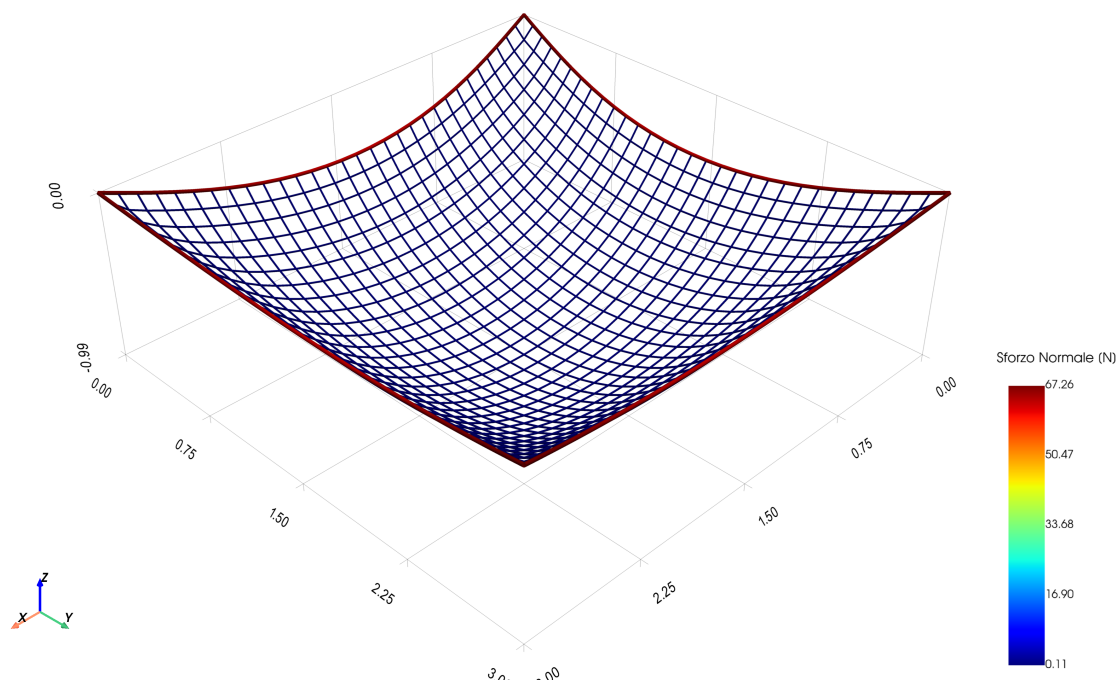
Figura 4.5: Rete vincolata ai nodi d'angolo
