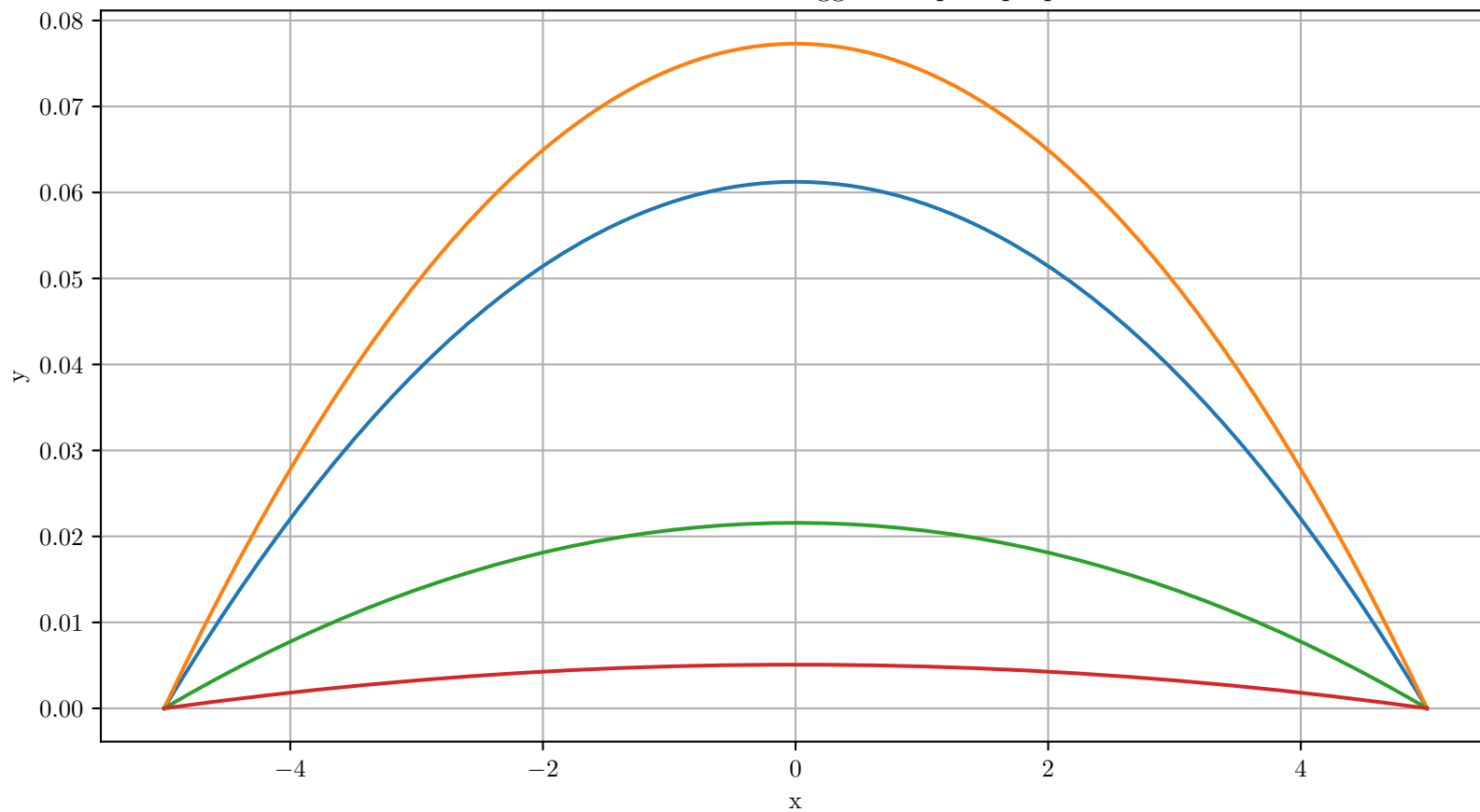
Deformate di funi tese soggette al peso proprio
