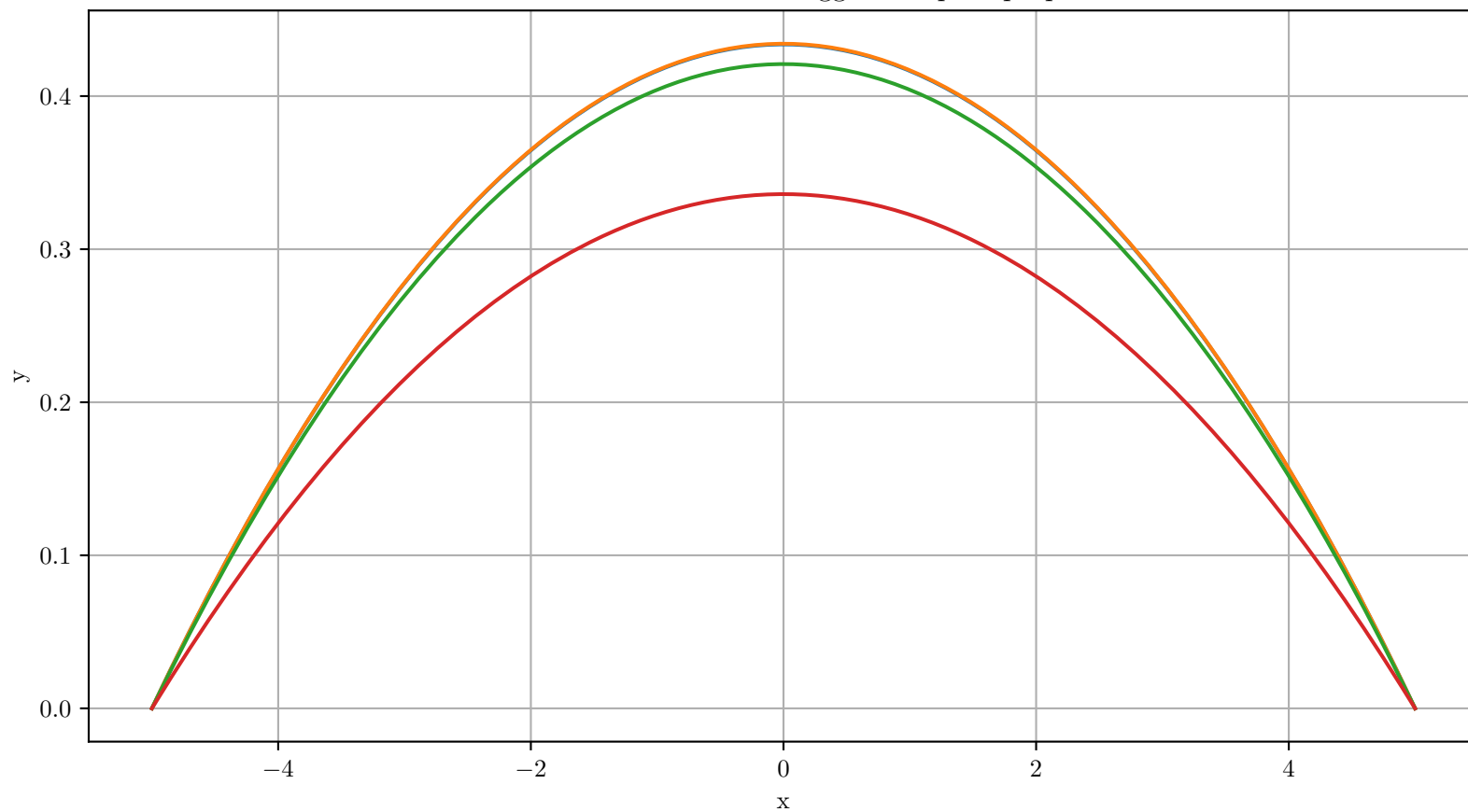
Deformate di funi lasche soggette al peso proprio
