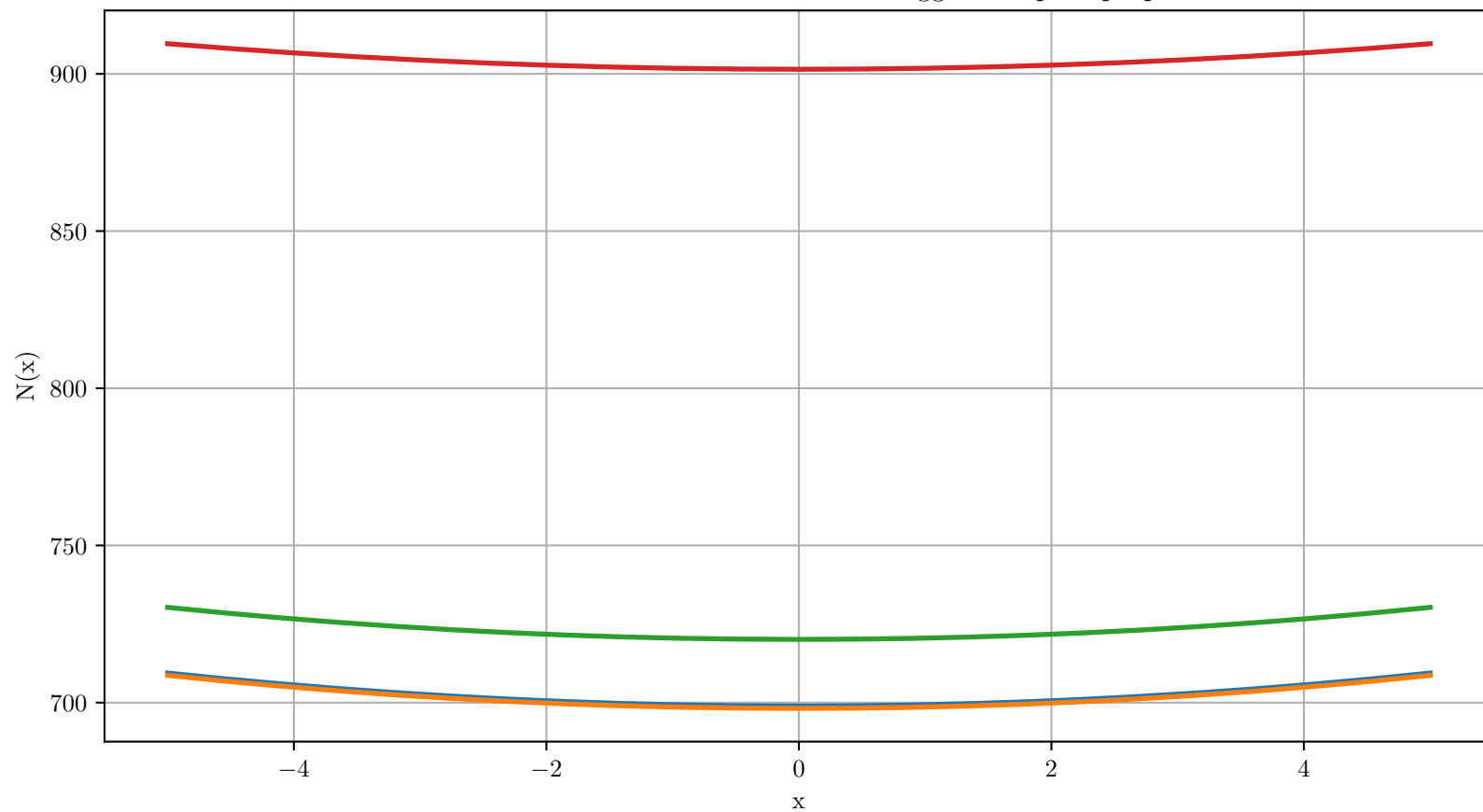
Sforzo normale nel caso di funi lasche soggette al peso proprio
