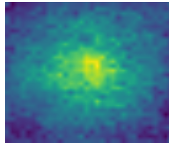
Layer 15
